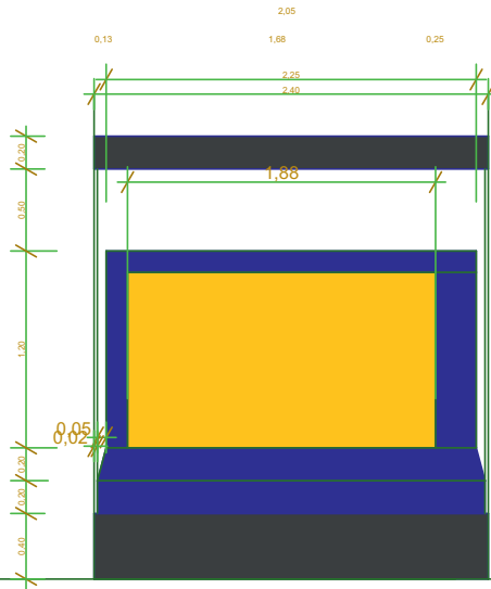
ΟΨΗ
